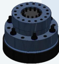
Platos cilíndricos para ensayos de alta carga. Hasta 50MN. Rocas, Metales
