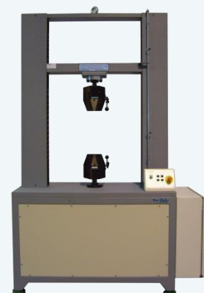
ME 405 + MORDAZAS DE TRACCION ACCIONAMIENTO MANUAL SERIE 4012
